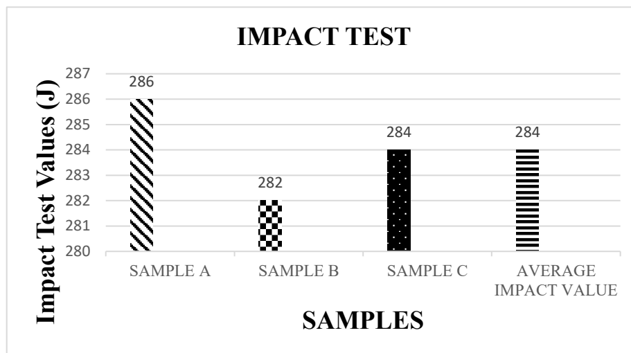
Fig. 18. Impact test chart.
